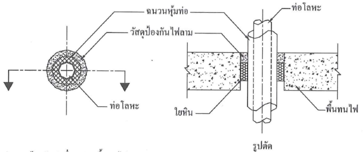
ตัวอย่างการป้องกันท่อนอื่น ๆ ผ่านพื้นทึนไฟ
