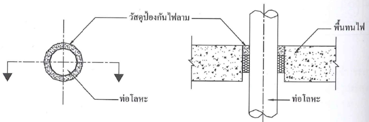
ตัวอย่างการป้องกันท่อโลหะผ่านพื้นทึบไฟ
