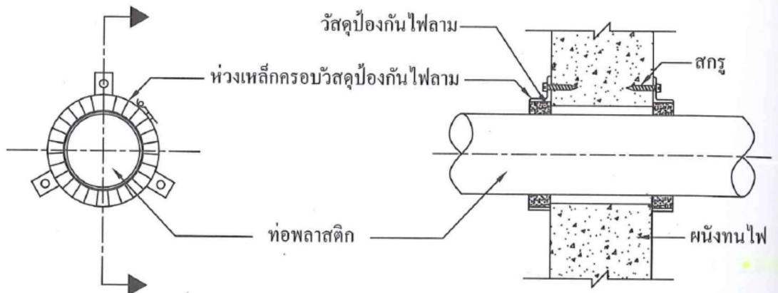
ตัวอย่างการป้องกันท่อพลาสติกผ่านผนังทึบไฟ
