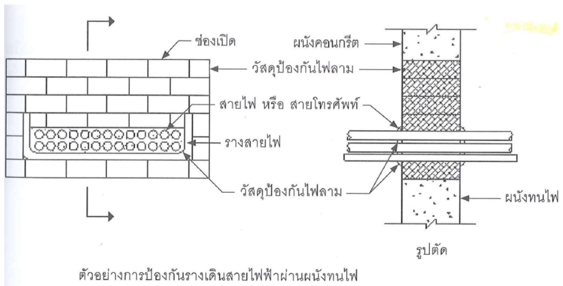
รูปที่ 2.6.5 การป้องกันรางเดินสายไฟฟ้าผ่านผนังท่อนไฟ
