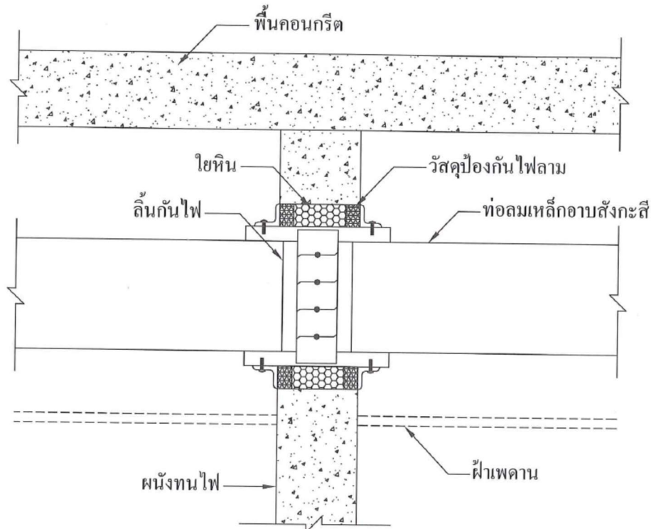
รูปที่ 2.6.3 การป้องกันท่อลมที่ไม่ได้ใช้งานผ่านผนังทนไฟขณะเกิดอัคคีภัย
